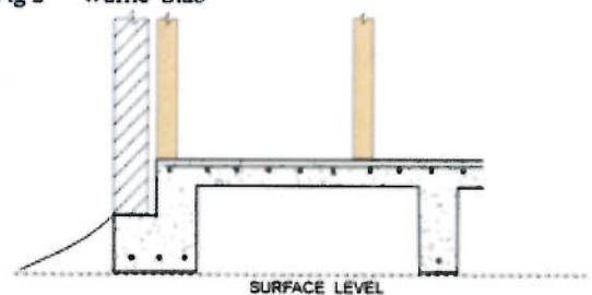
Fig 2 Waffle Slab
